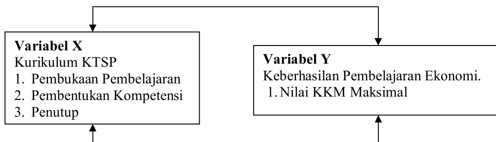
Gambar 1.1 Kerangka Pemikiran
